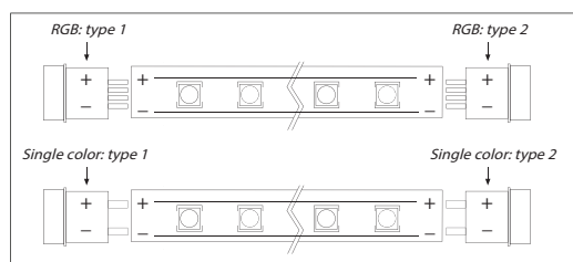
Aansluitsnoer types Types de câbles de connexion
