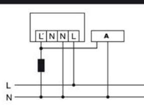
Bij schakeling van inductoren (bijv. relais, magneetschakelaars, voorschakelapparatuur) kan een RC-filter (A) nodig zijn.
