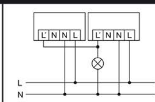
Parallelschakeling van max. 8 apparaten
