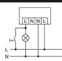
Standaardschema met extra continulichtfunctie via externe schakelaar.
