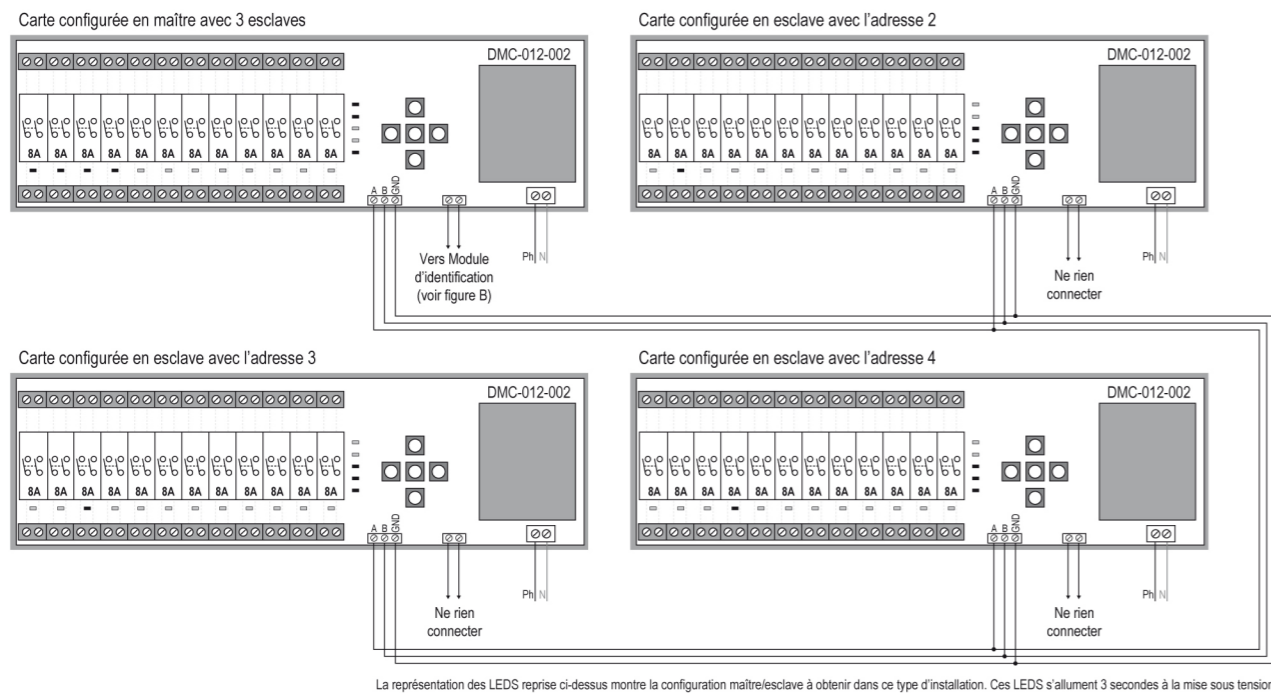
La représentation des LEDS reprise ci-dessus montre la configuration maître/esclave à obtenir dans ce type d'installation. Ces LEDS s'allument 3 secondes à la mise sous tension.
