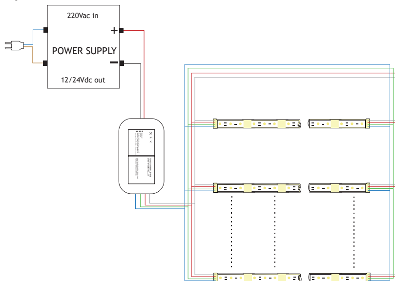
Aansluitschema Base drawing
