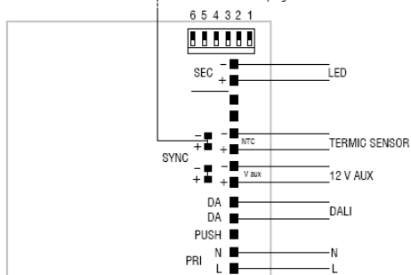
Schema collegamento con segnale DALI Wiring with DALI signal
