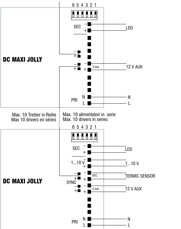
Schema con 1...10 V o potenziometro - Diagram with 1...10 V or potentiometer - Diagramm mit 1...10 V oder Potentiometer - Schéma avec 1 ... 10 V ou potentiomètre
