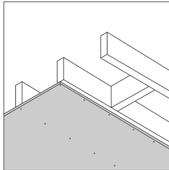
Gipsplaat
