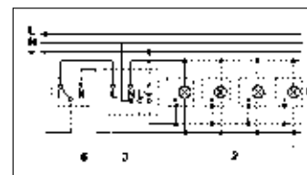
4. Allacciamento tramite deviatore uso d'operazione automatico e ad illuminazione permanente
