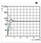
CDM-TC 20W /830 + Zoom
